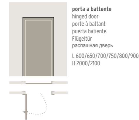
con telaio esterno with external frame avec châssis extérieur con marco exterior mit Außenrahmen с наружной направляющей
