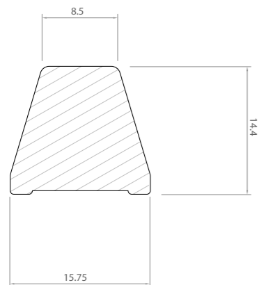
1. traverso verticale vertical crosspiece | traverse verticale | travesaño vertical vertikale Traverse | вертикальная рейка
